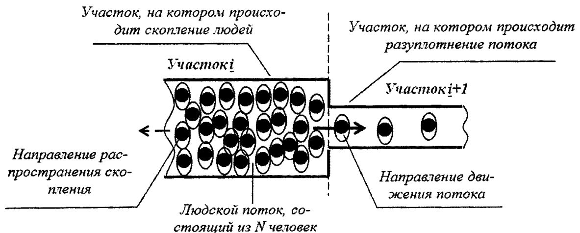
Рисунок Пб.1. Пояснения к расчету параметров людского потока
